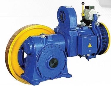
Asenkron Dişlili Motor Asynchronous Geared Motor
