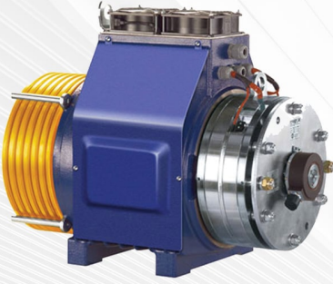
Senkron Dişlisiz Motor Asynchronous Gearless Motor
